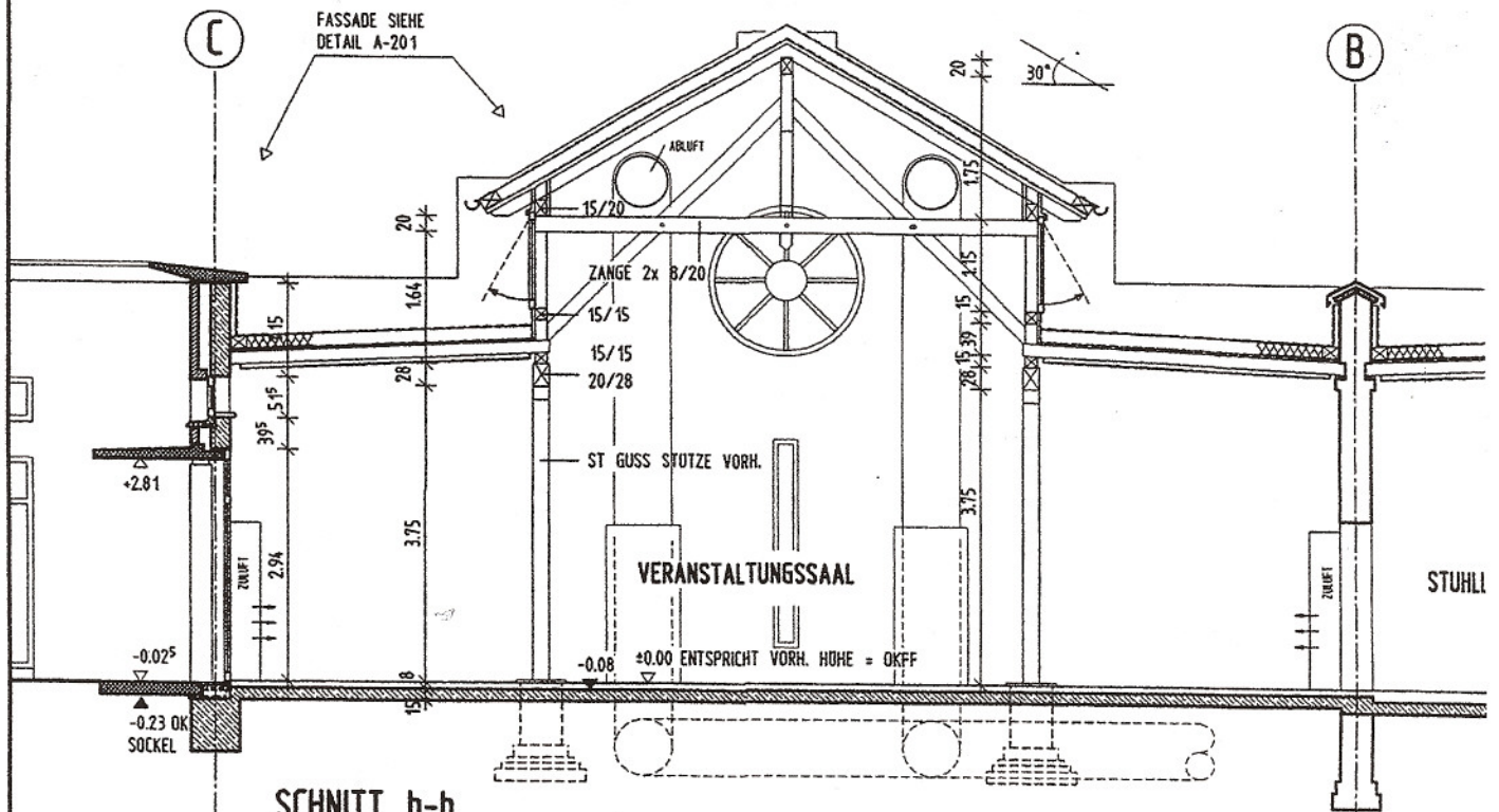
SCHNITT b-b
